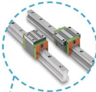
Роликовые линейные направляющие HIWIN/PMI (Тайвань)
