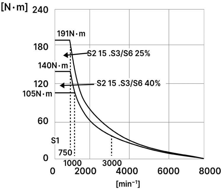
ДИАГРАММА МОЩНОСТИ / КРУТЯЩЕГО МОМЕНТА / ЧАСТОТЫ ВРАЩЕНИЯ ДВИГАТЕЛЯ FANUC
