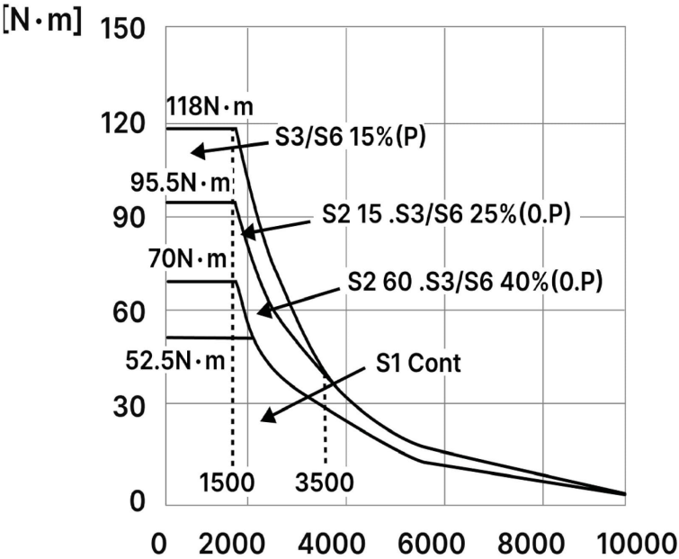
ДИАГРАММА МОЩНОСТИ / КРУТЯЩЕГО МОМЕНТА / ЧАСТОТЫ ВРАЩЕНИЯ ДВИГАТЕЛЯ FANUC
