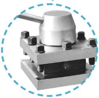
Резцедержатель (25x25 мм, поворот ±90°)
