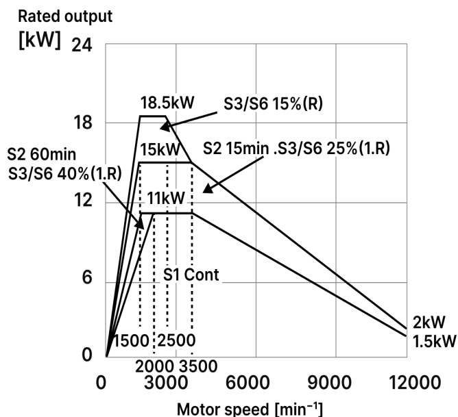
Диаграмма мощности/крутящего момента/частоты вращения двигателя Fanuc
