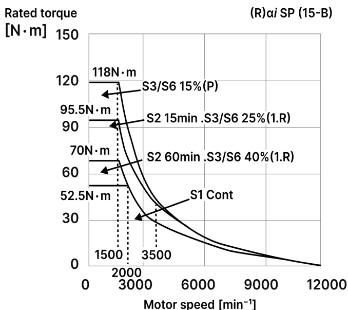
Диаграмма мощности/крутящего момента/частоты вращения двигателя Fanuc
