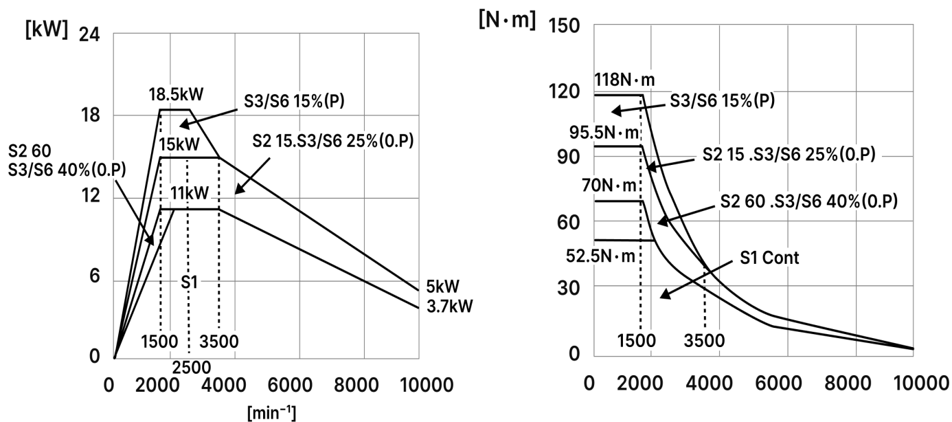
Диаграмма мощности/крутящего момента/частоты вращения двигателя Fanuc
