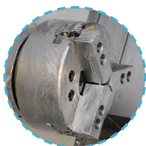
Трехкулачковый токарный патрон
