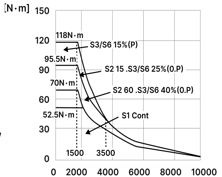
Диаграмма мощности/крутящего момента/частоты вращения двигателя Fanuc
